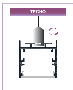
② Poner el perfil y enroscar el anclaje para sujetarlo
