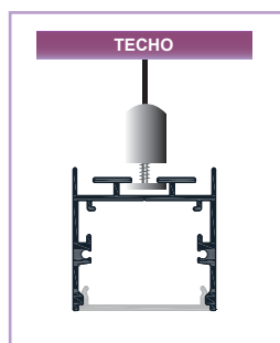
① Colgar el cable con el aplique sin enroscar
