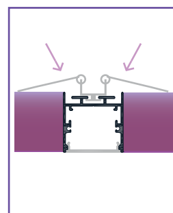
③ Dejar caer las aletas de las pinzas al empotrarlo y encajar el perfil
