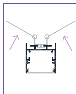
② Abrir las aletas de las pinzas para empotrarlo
