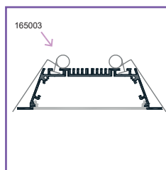
① Colocar las grapas en los laterales del perfil
