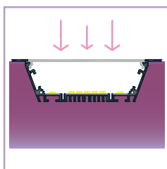
③ Encajar el difusor en el perfil
