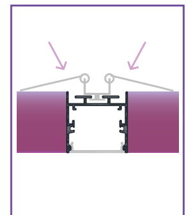
③ Dejar caer las aletas de las pinzas al empotrarlo y encajar el perfil
